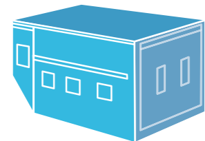
ENVASE EN BAJO CUBIERTA - IATA TIPO 8 - IATA PREFIJO: AK - ATA: LD-3
